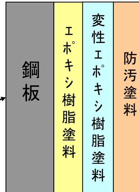
船底部の断面
