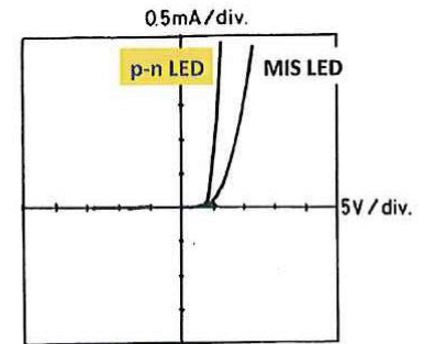
GaN LEDの電流-電圧特性
